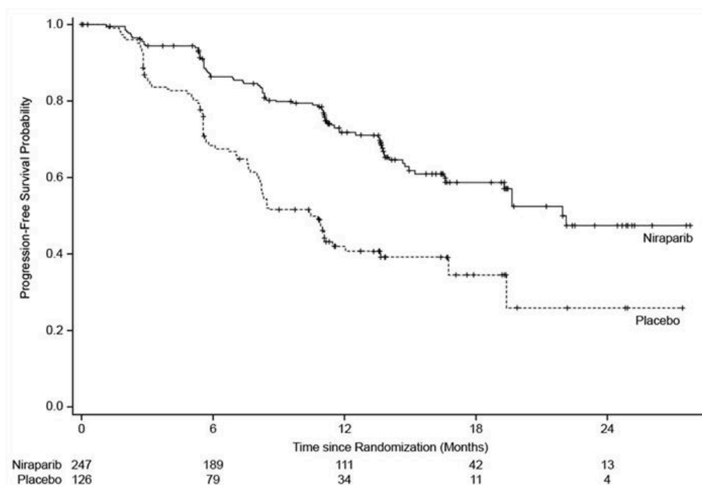
圖 2：整體族群的無惡化存活期－PRIMA (意圖治療群體，N=733)
