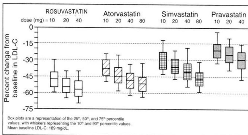
圖1. 第6週時ROSUVASTATIN、Atorvastatin、Simvastatin及Pravastatin劑量在高脂血症或混合型高脂血症病人中造成的低密度脂蛋白膽固醇百分比變化
